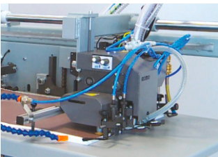
Cabezal mecánico (sólo modelo TF)
